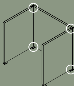
Samlebeslag artikelnr. 5221
