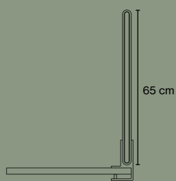
Klemmebeslag artikelnr. 3029
