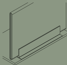
Fristående hållare artikelnr. 3033
