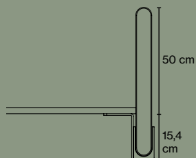
Frontmonterat beslag artikelnr. 5032
