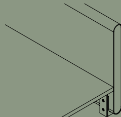
Frontmonteret beslag artikelnr. 5032
