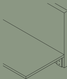
Frontmonterat beslag artikelnr. 3040
